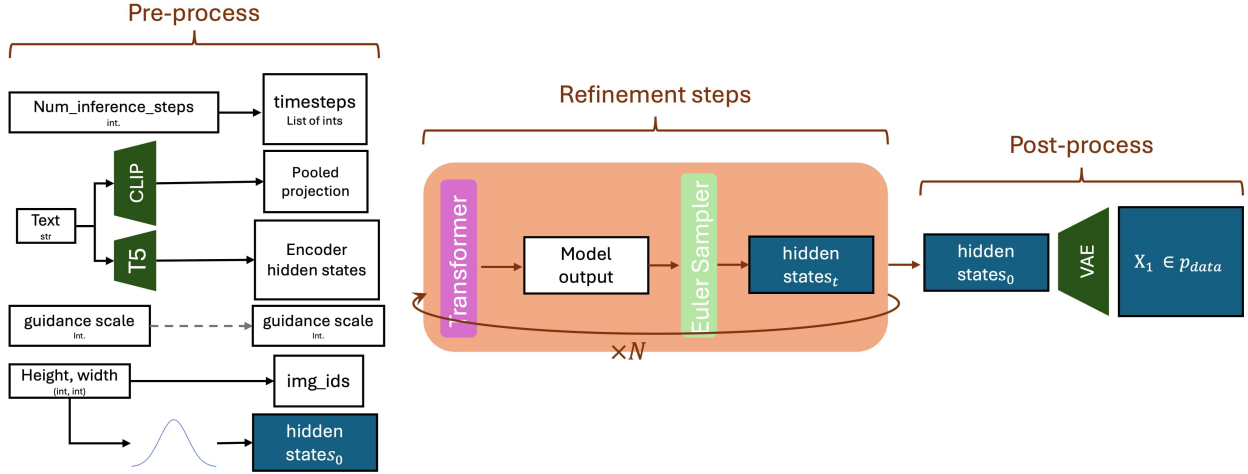
图 5: Flux.1 采样流水线。与扩散模型一样，预处理之后，含噪潜在变量 z_t （记为 hidden\_state_t ）在潜在空间中被迭代精修。最终精修得到的 z_0 ( =hidden\_states_0 ) 经预训练的 VAE 解码器解码为 RGB 图像。
