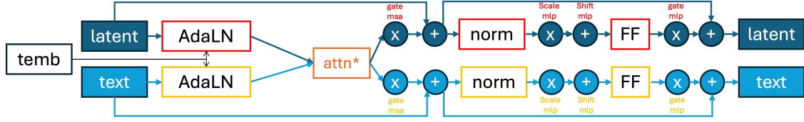
(a) 双流注意力块：潜在嵌入与提示词嵌入分别处理，采用标准的多模态注意力方案。
