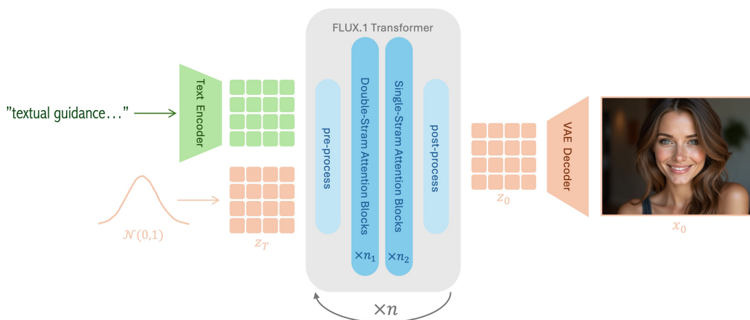
图 4: FLUX.1 架构的高层概览。文本嵌入与潜在图像嵌入经由一系列注意力块被迭代处理，从而生成文本条件下的图像。
