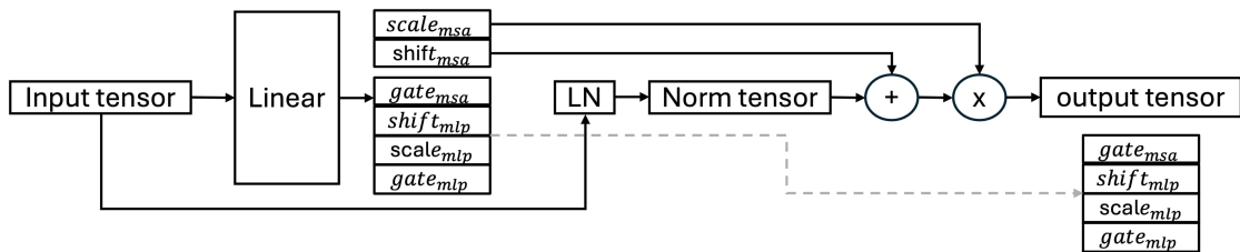
图 9: AdaLN 层, 其中 MSA (多头自注意力, Multi-head Self Attention) 与 MLP (多层处理器, Multi-Layer Processor) 的调制参数根据输入张量计算。在单流块 (见 节 2.3.3) 中不计算 MLP 调制。
