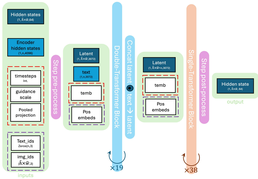
图 6: Flux Transformer: 高层概览
