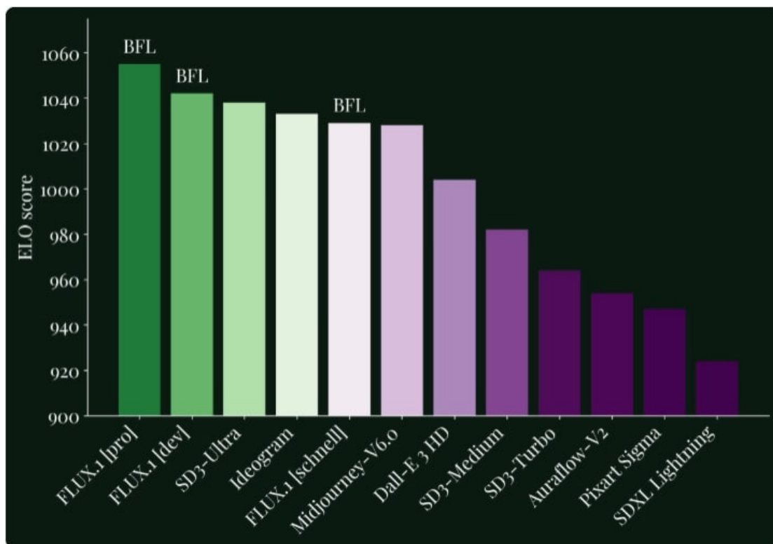
图 2: 在文生图合成中, FLUX.1 在图像细节、提示词遵循度、风格多样性与场景复杂度上重新定义了最先进水平。评测数据来自 [18]。
