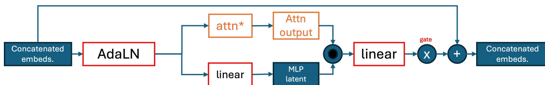
(a) 单流注意力块：潜在嵌入与提示词嵌入一起处理，采用同时进行的注意力方案。
