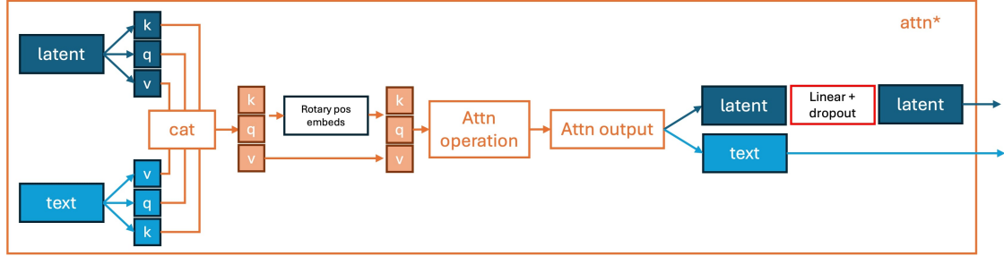
(b) 注意力操作施加于拼接后的 token 上。
