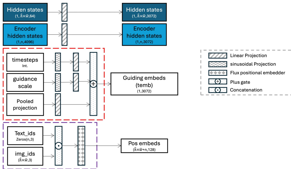
图 7: Flux Transformer: 每次迭代的输入预处理
