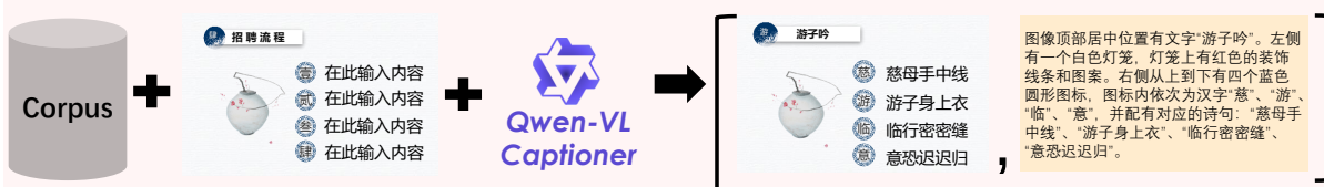
图 13: 数据合成概览。我们设计了三种渲染策略——纯渲染（Pure Rendering）、组合渲染（Compositional Rendering）和复杂渲染（Complex Rendering）——分别用于生成纯文本数据、文本上下文数据和复杂布局数据。
