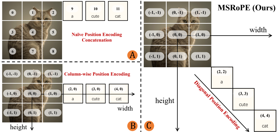
图 8: 不同图像-文本联合位置编码策略的比较。我们提出的多模态可扩展 RoPE (MSRoPE) 策略从图像中心开始编码, 将文本编码沿网格对角线定位, 实现更好的图像分辨率缩放和改进的文本-图像对齐。
