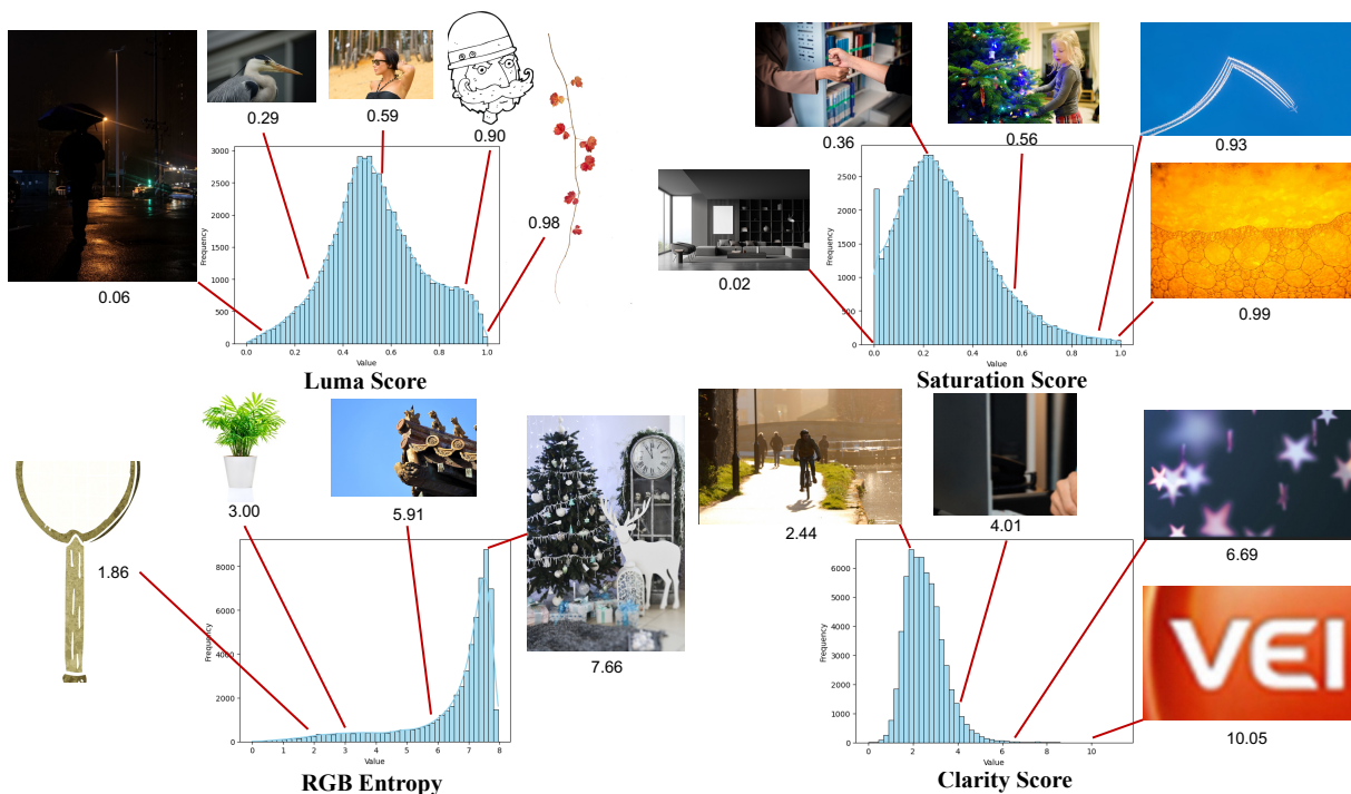
图 11: 流水线中使用的某些过滤算子的示例。这些算子中的极值通常表明非典型或低质量图像。例如，Luma 分数过高的图像通常包含大范围白色或曝光过度的区域。
