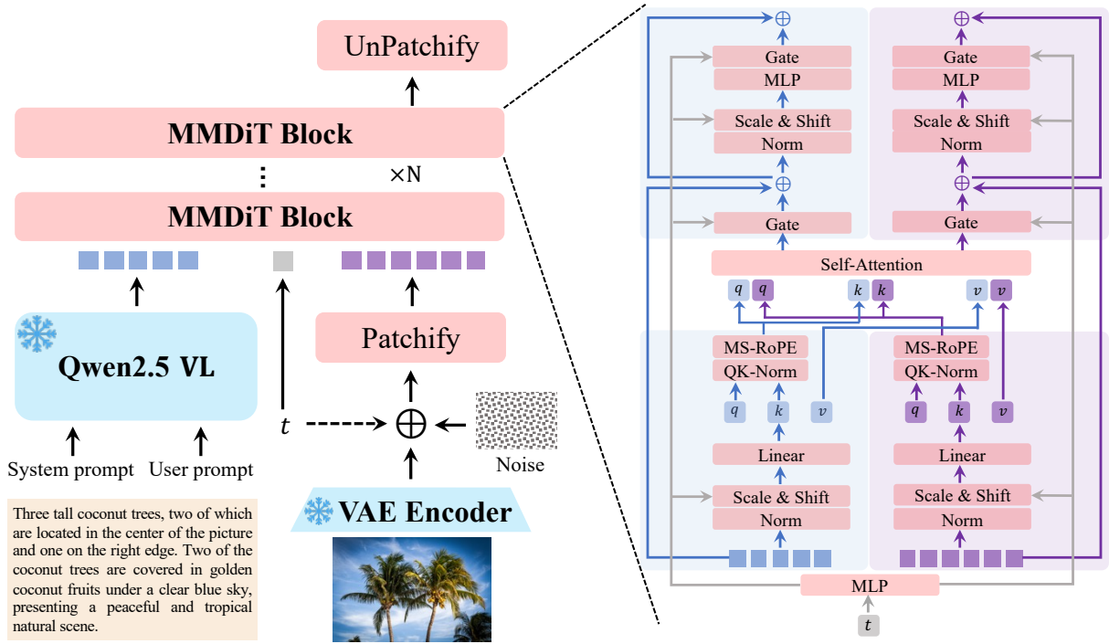
图 6: Qwen-Image 架构概览。采用标准双流 MMDiT 架构。输入表示来自冻结的 Qwen2.5-VL 和 VAE 编码器。QK-Norm 采用 RMSNorm (Zhang & Sennrich, 2019)，其他规范化层采用 LayerNorm。新设计的位置编码方案 MSRoPE（多模态可扩展 RoPE）联合编码图像和文本模态的位置信息。
