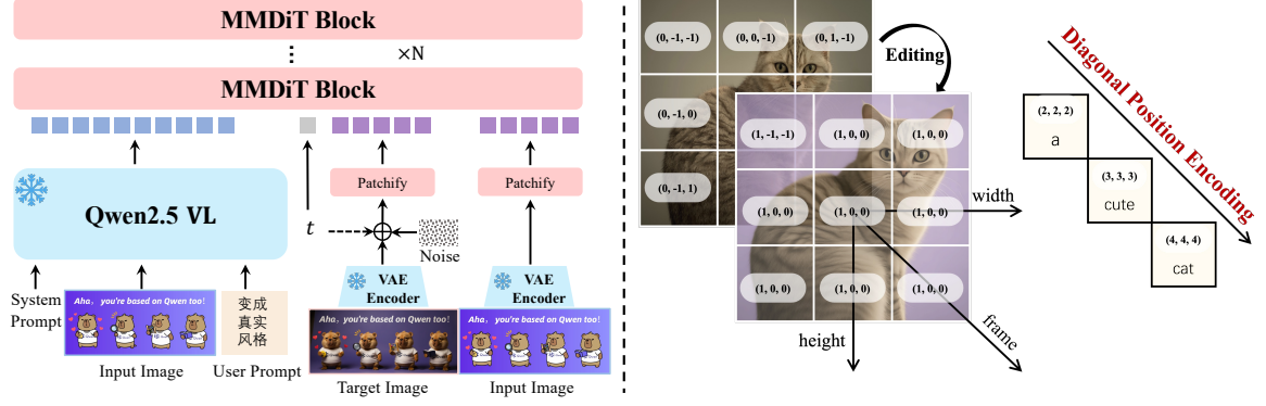
图 14: 图像编辑 (TI2I) 任务概览。左图: TI2I 任务训练输入格式的示意图。用户提示为英文”Turn into realistic style”。右图: TI2I 对应的 MSRoPE 修改, 引入新的维度 (帧) 以区分编辑前后的图像。
